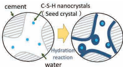
図 1 強度発現改善のメカニズム
