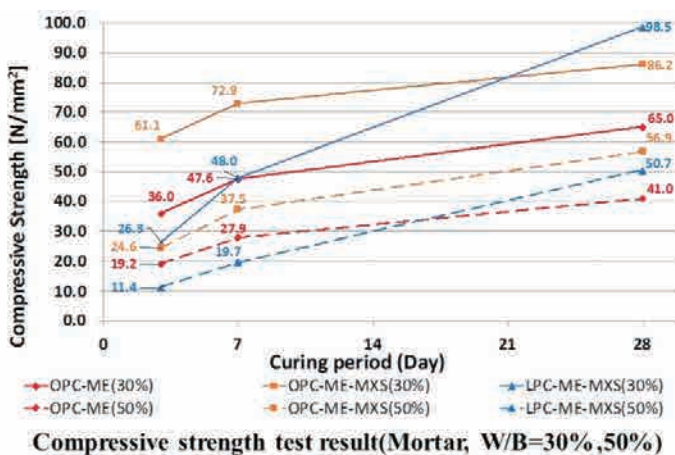
図 2 各配合の圧縮強度試験結果
