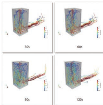
八戸工業大学地域産業総合研究所によるBOXer TYPE.1（隣）開発時の空調シミュレーション
